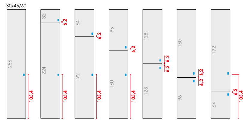
Schema maniglie passo 9,6 Pitch 9.6 handles diagram
