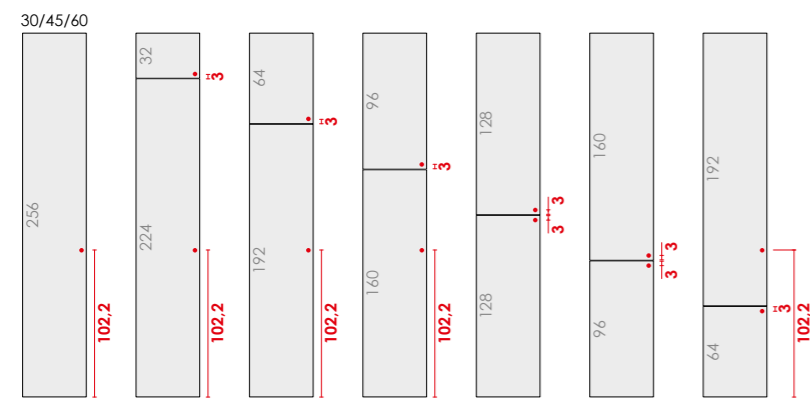
Schema maniglie passo 3,2 Pitch 3.2 handles diagram
